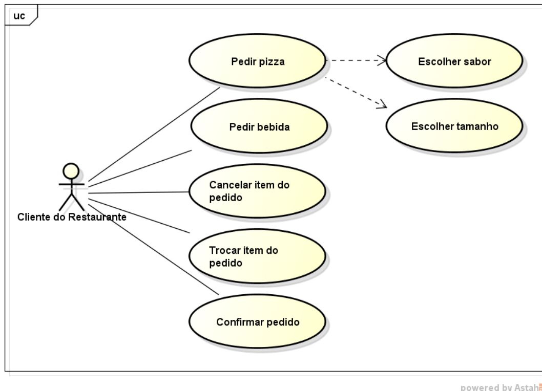
Figura 7: Diagrama de casos de uso relativo ao projeto. Autoria própria.
